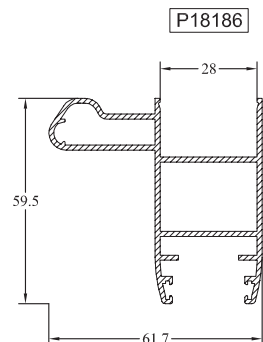
Montant serrure renforcé
