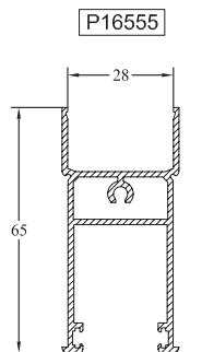
Traverse haute et basse
