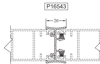
Chicane bout à bout
