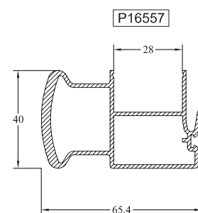
Montant chicane renforcé
